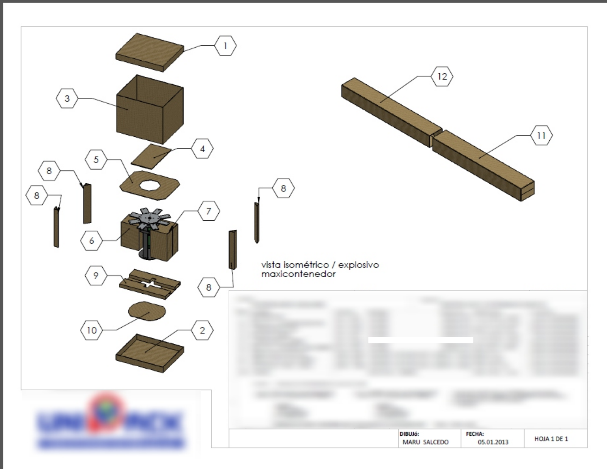
Contenedor para ventilador industrial.
