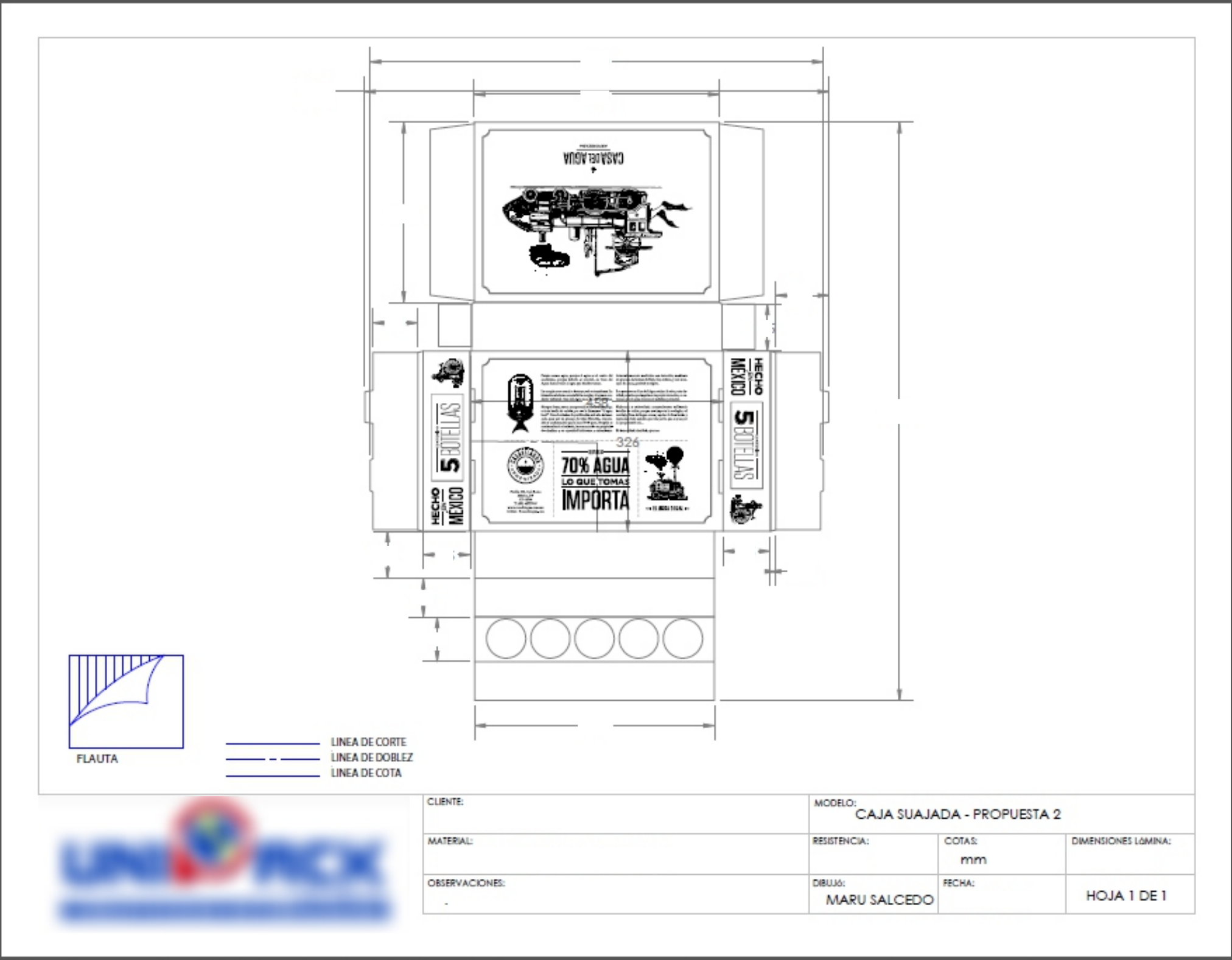
Empaque para botellas de agua.
